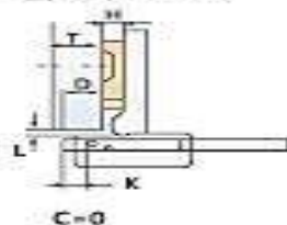
盖位公式 H=12+K-D
